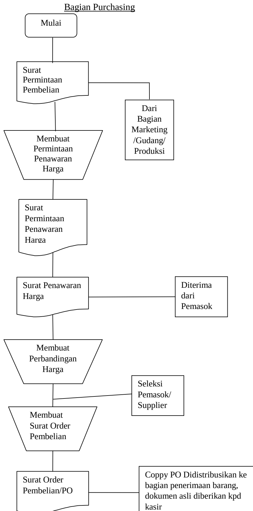
Gambar 4.2 Flowchart Prosedur Sistem Akuntansi Pembelian pada PT Gramaselindo Utama
