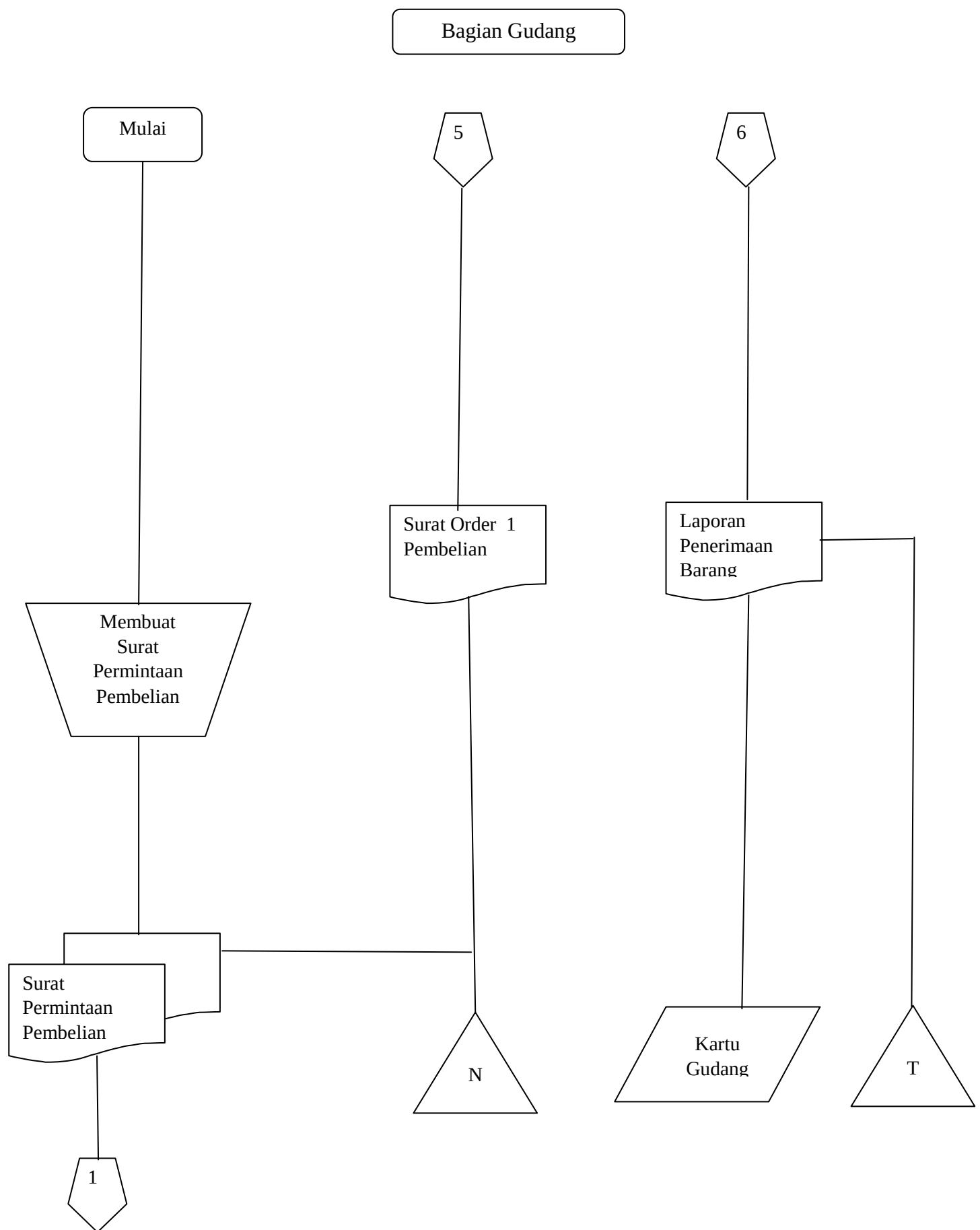
Gambar 2.2 Flowchart Sistem Akuntansi Pembelian
